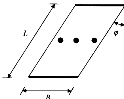
Figura 7.9.1 - Ponte obliquo
